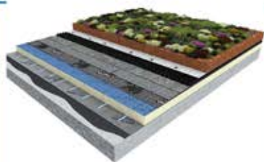
Gründachaufbau: Komplett aus einer Hand vom Voranstrich bis zur Begrünung
